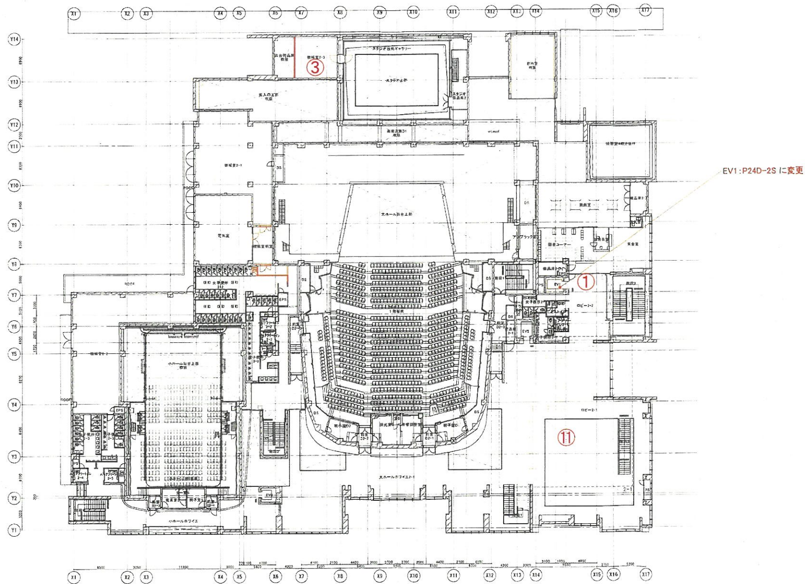
変更後 2F平面図 1:400
