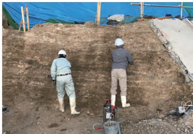
盛土の構造を復旧に生かすために、石垣背後の盛土層を確認している様子(3月上旬)
