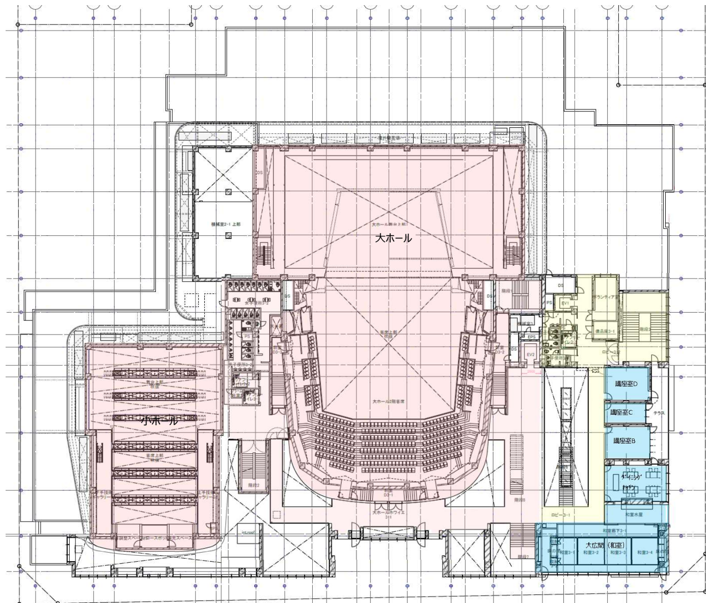
施設内諸室配置案 3階平面図
