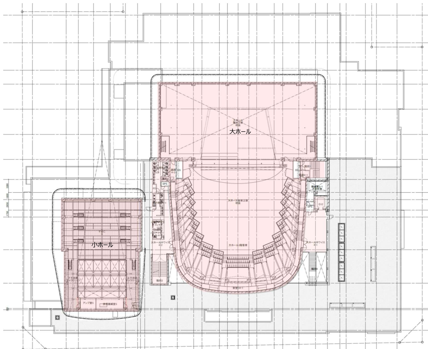
施設内諸室配置案 4階平面図
