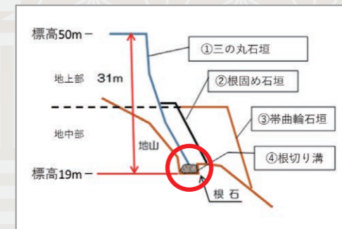
石垣の基礎構造
