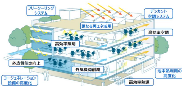
ZEB の概要（出典：資源エネルギー庁資料）
