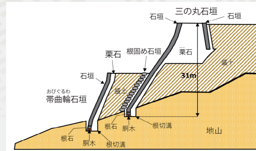
崩落前の姿(断面図)
