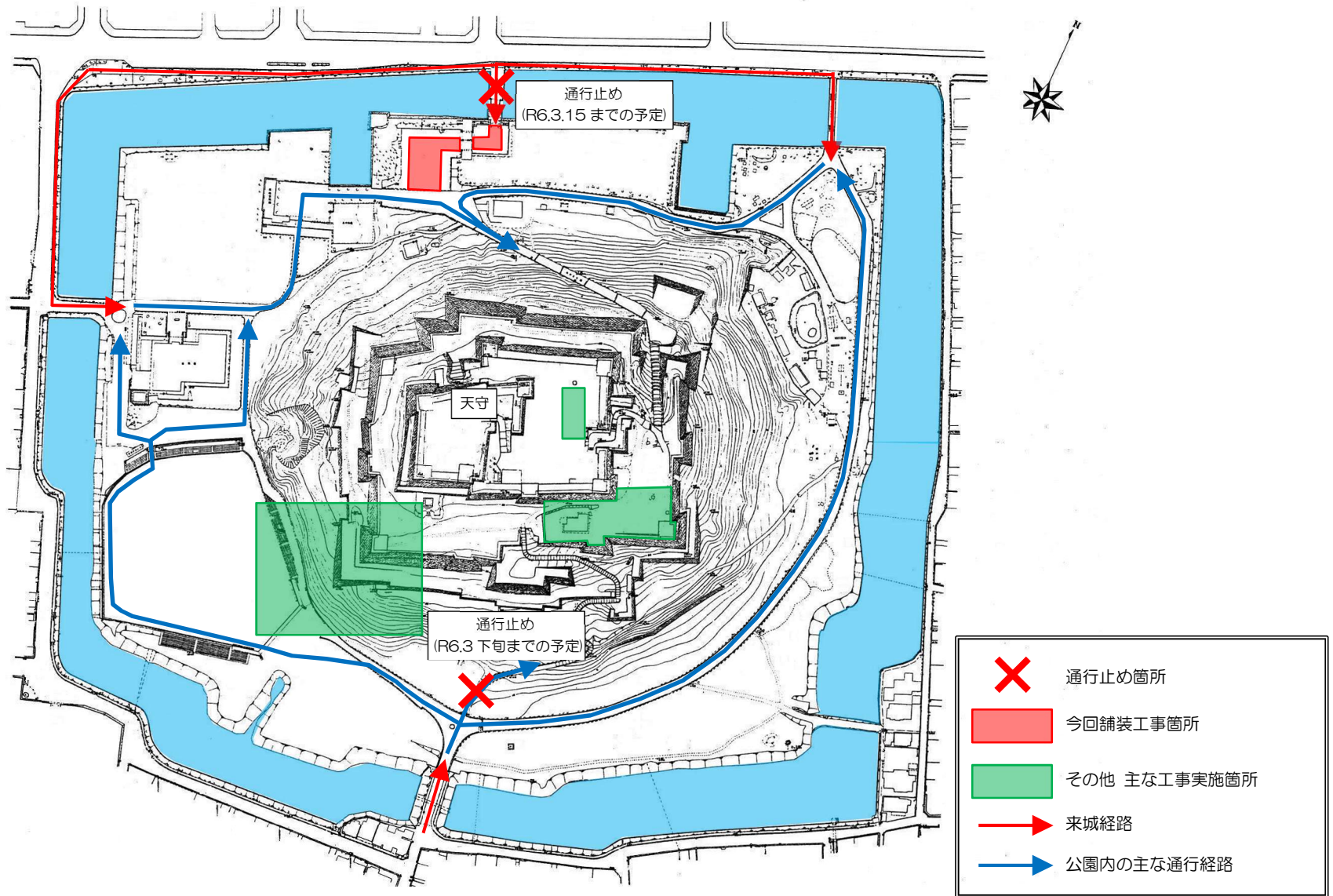
史跡丸亀城跡平面図 0 100M
