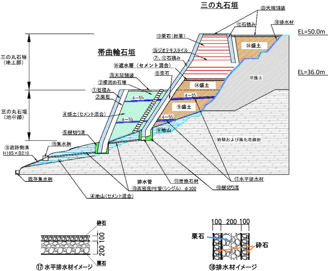
石垣断面図（現代工法採用）
