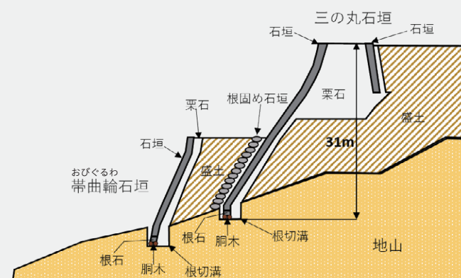
崩落前の姿(断面図)
