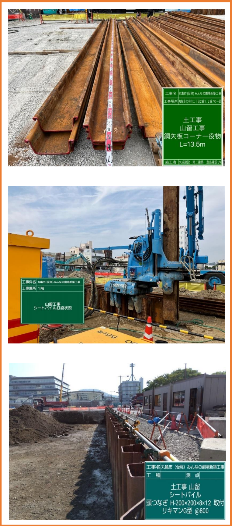
仮設土留板(シートパイル)施工状況
