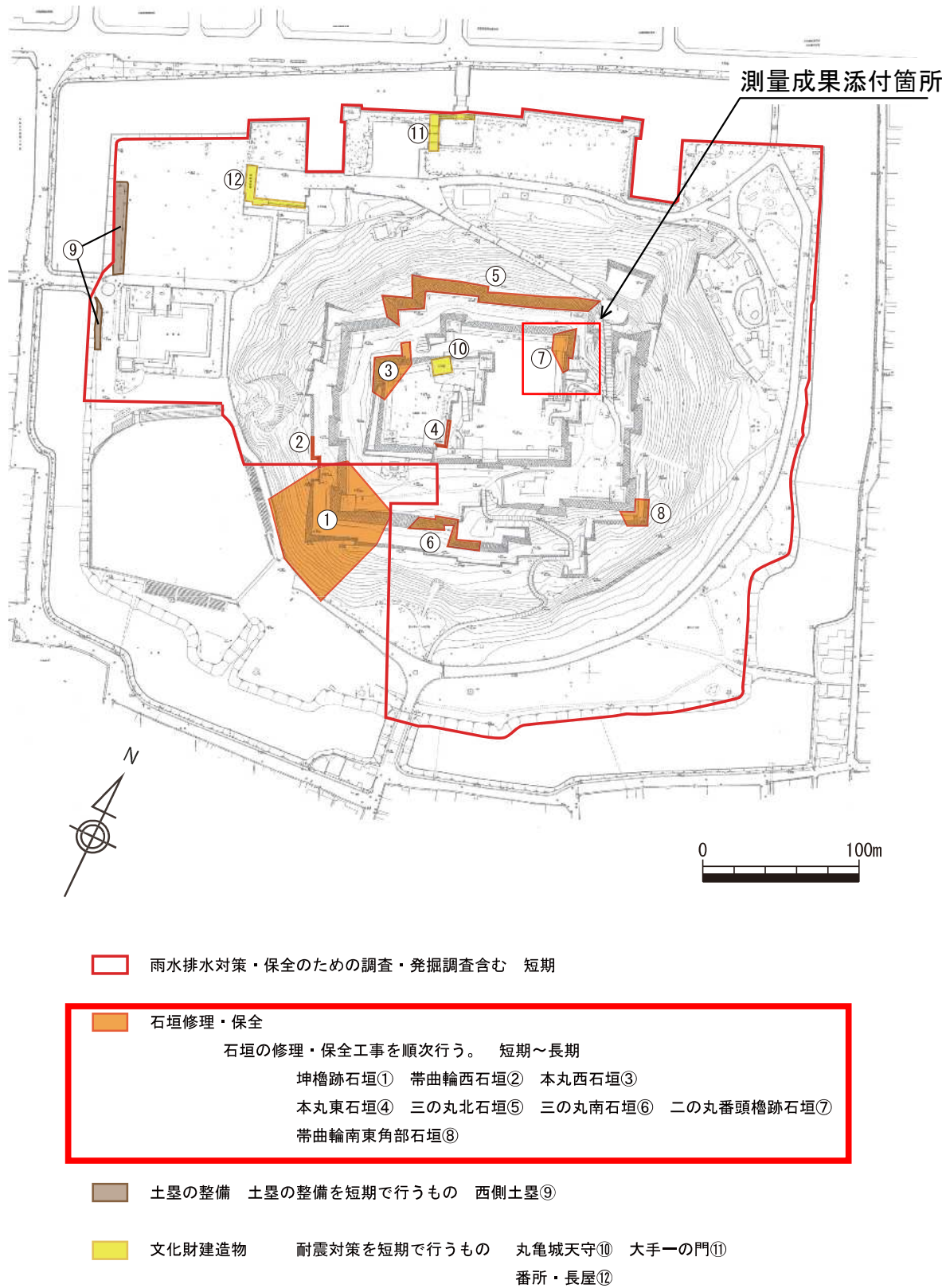
図 41 保存のための整備
