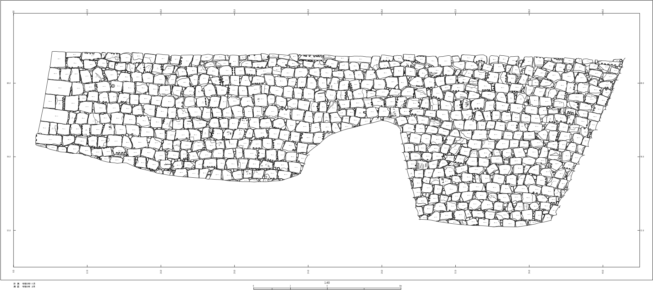
史跡丸亀城跡二の丸東側石垣 69 立面図
