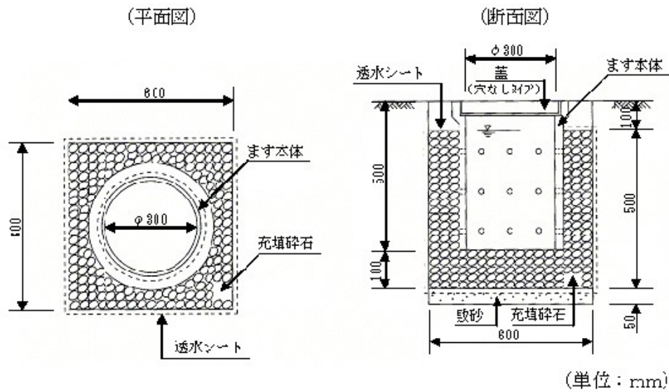
雨水浸透ます標準構造図
