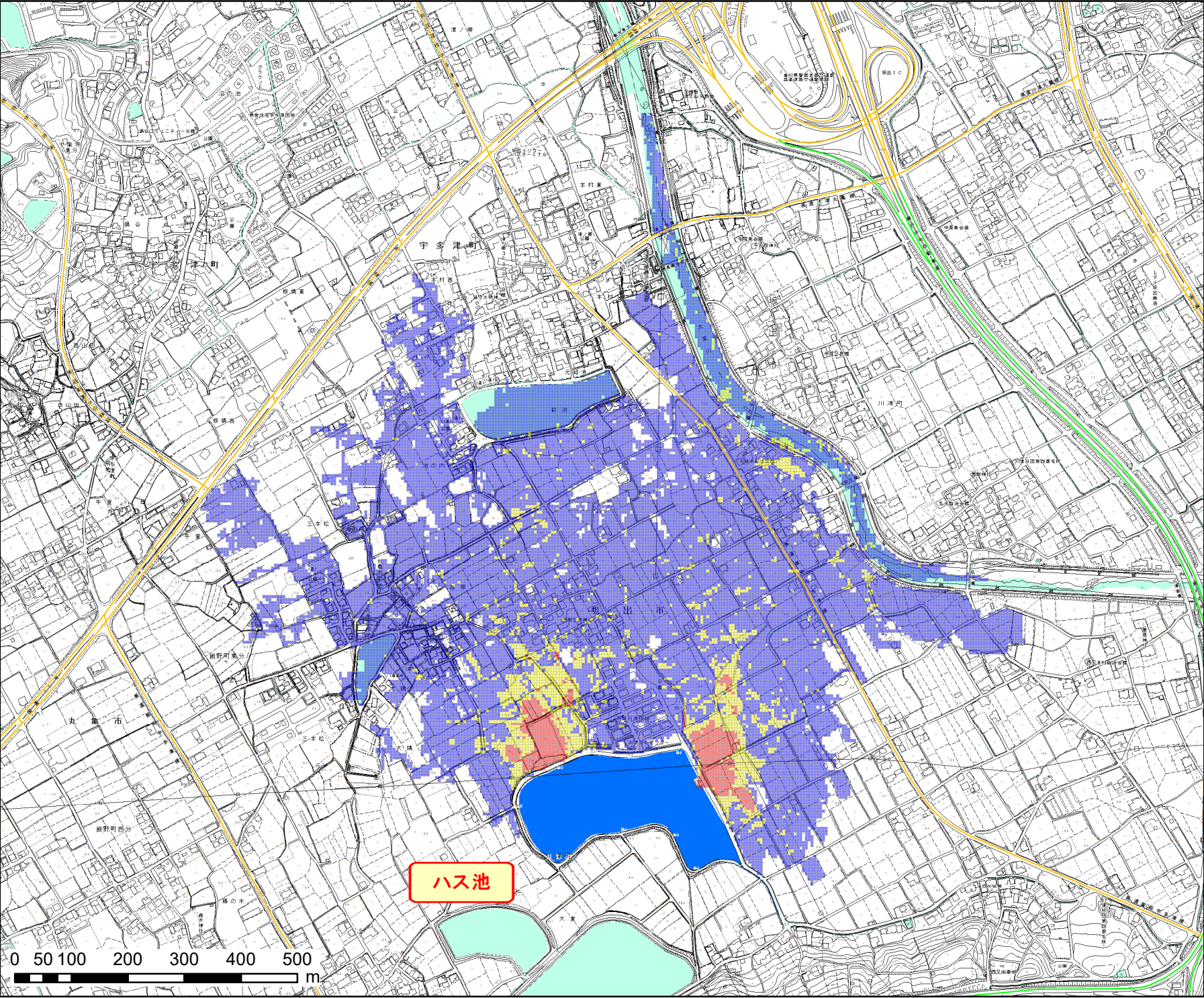
坂出市ため池氾濫解析 浸水想定区域図 (歩行困難度)
