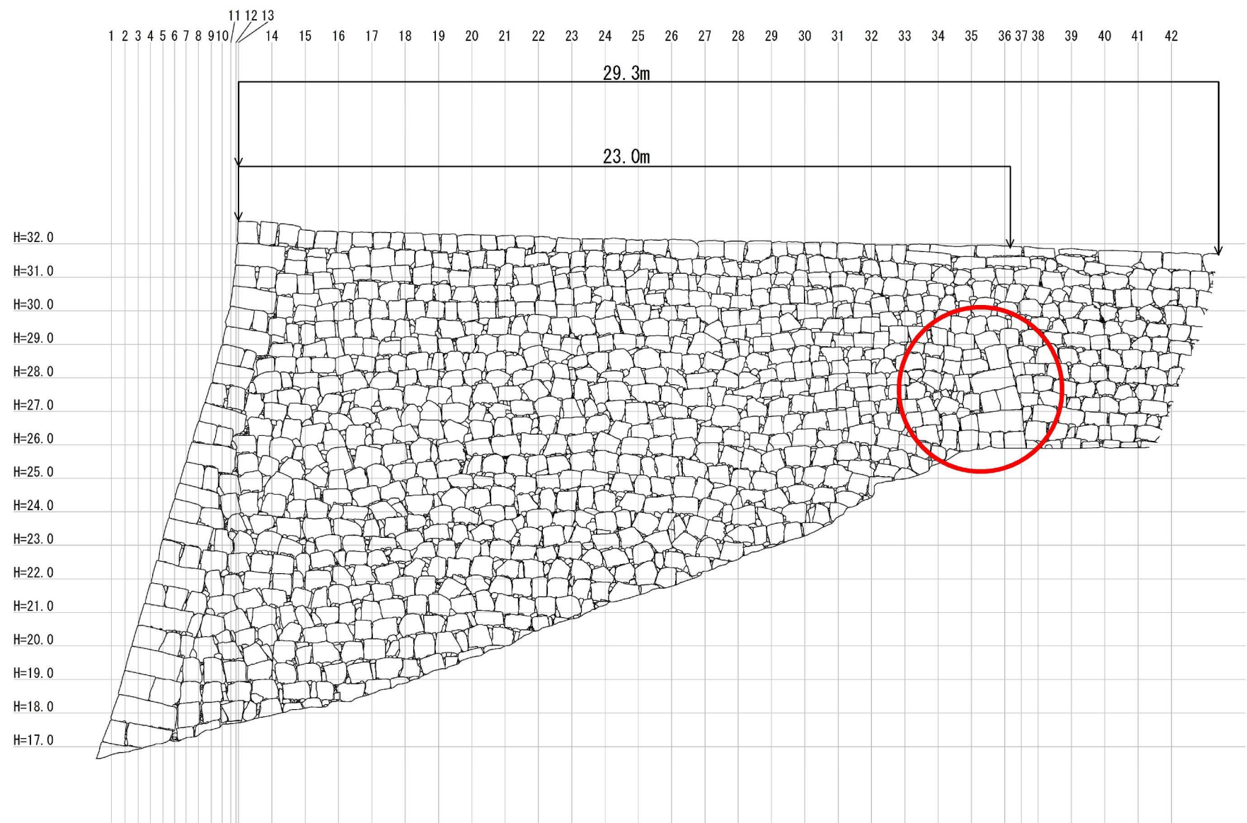
I 面立面図における算木積みの位置
