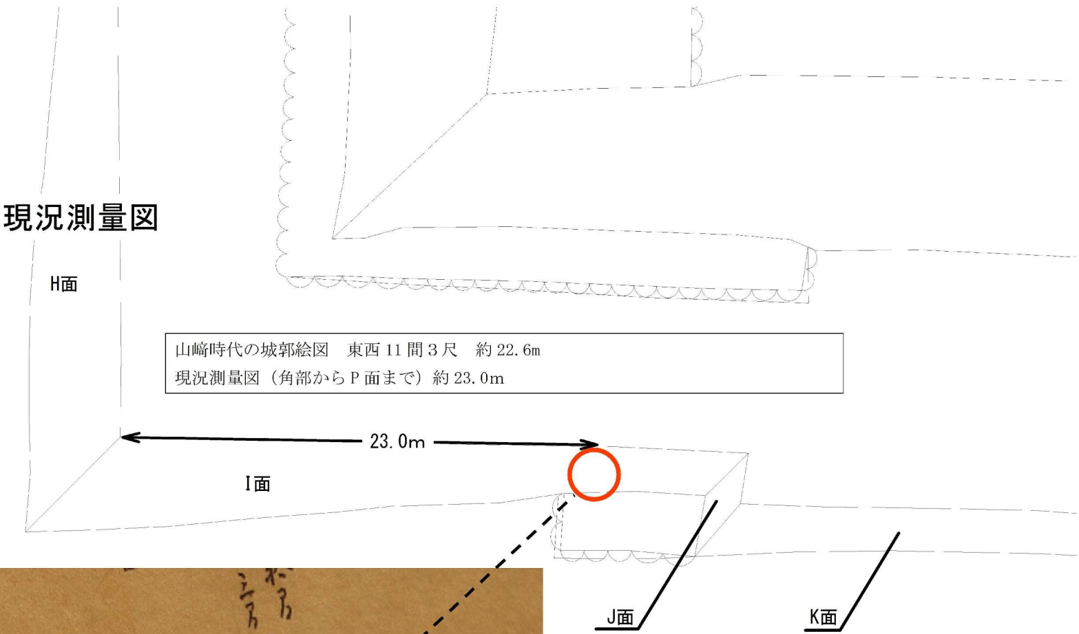
I 面立面図における算木積みの位置
