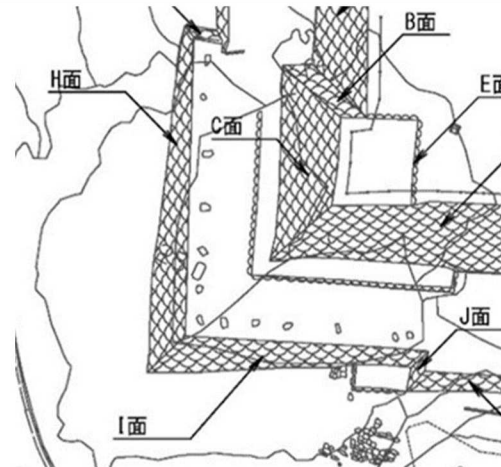
現況帯曲輪石垣（H面 I面位置）
