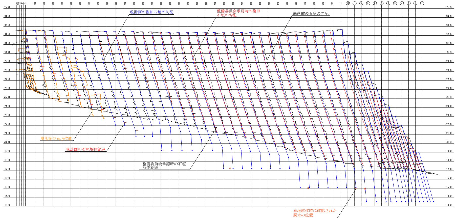
帯曲輪（H面） 集合断面図
