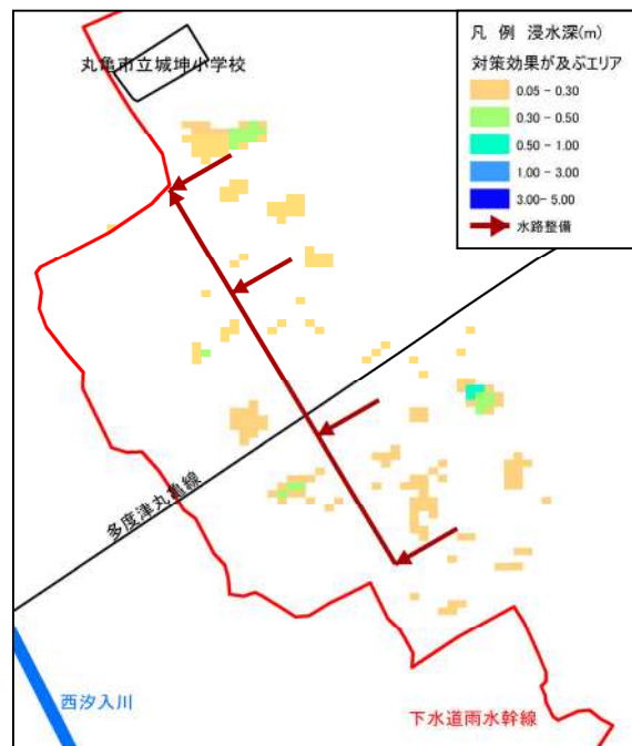
図 2.3.2 R4 洪水の降雨波形に基づく浸水予想図（対策後）
