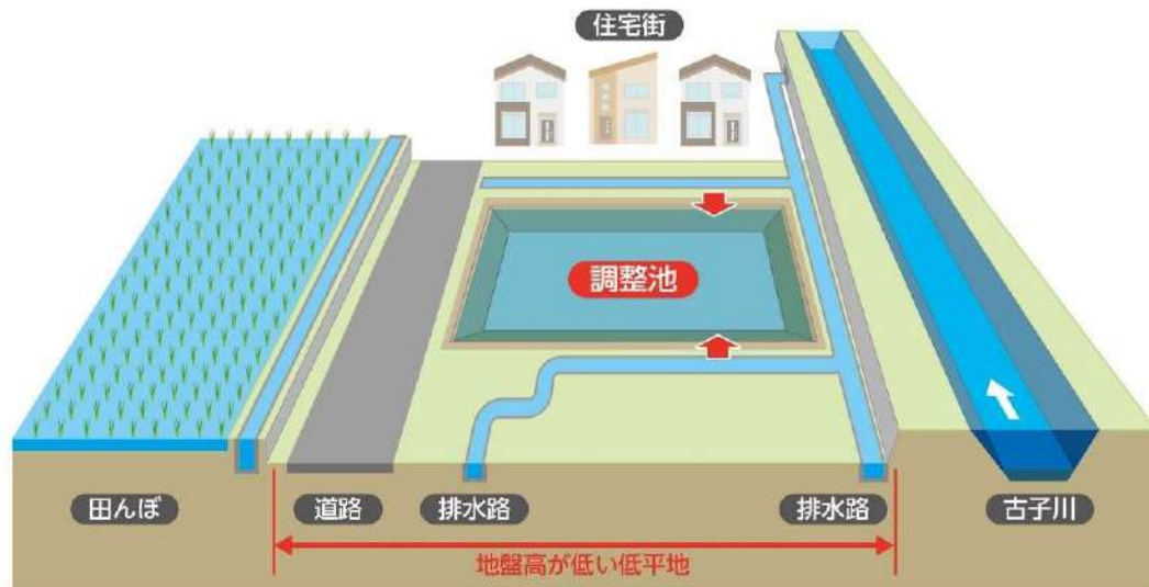
図 5.1.3 調整池による流出抑制対策のイメージ
