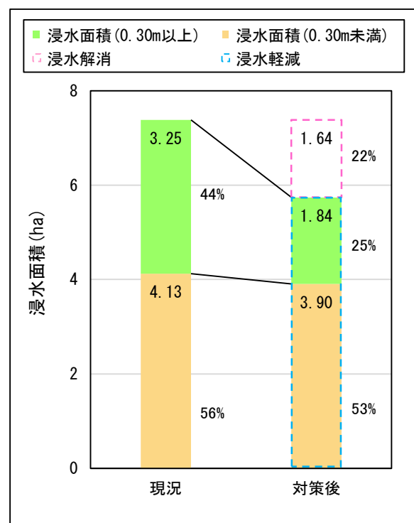
図 2.4.4 浸水面積の変化
