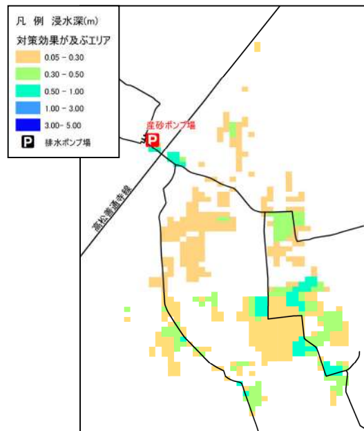
図 2.4.2 R4 洪水の降雨波形に基づく浸水予想図（対策後）
