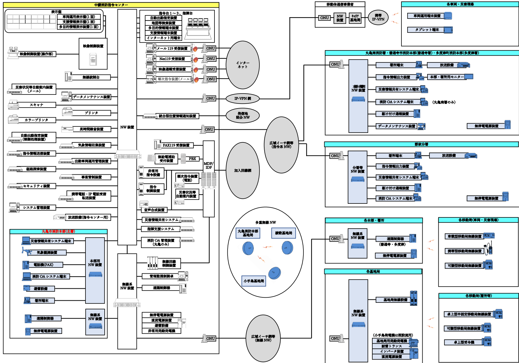
【別紙2】 システム全体構成図
