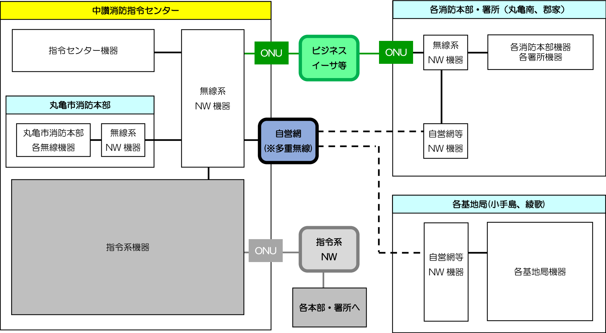
【別紙 11】 無線系ネットワーク構成図
